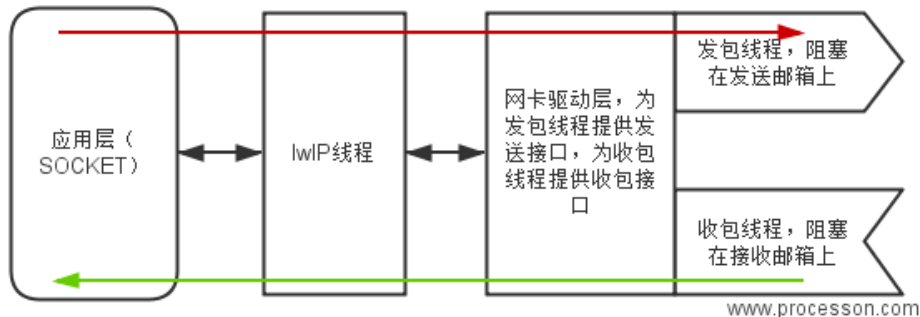
图 14.5: RTT收发包设计
