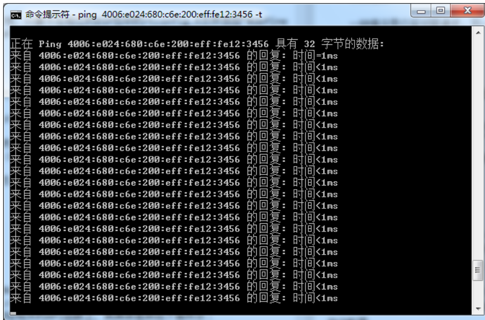
图 15.5: ping6
