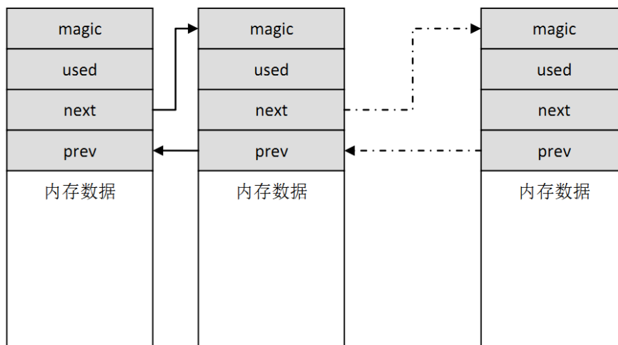
图 5.2: 内存块链表
