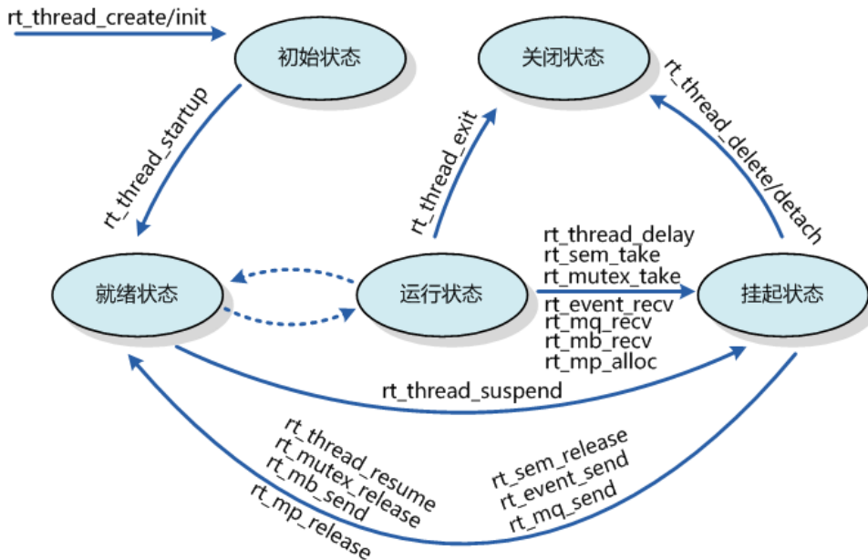
图 2.2: 线程转换图
