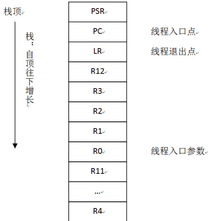
图 9.7: 堆栈压入情况图
