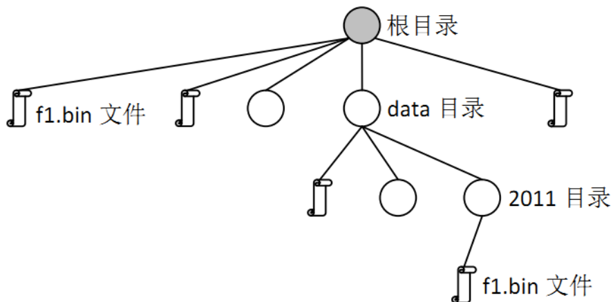
图 12.2: 目录结构
