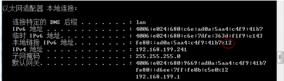
图 16.3: Scope ID
