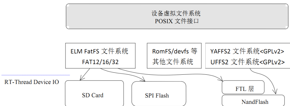
图 13.1: 文件系统结构图
