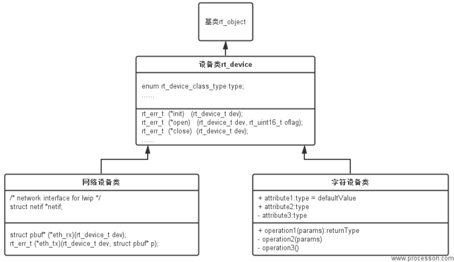
图 16.3: RTT设备继承关系
