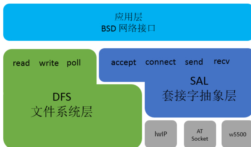
图 14.1: SAL 网络框架图
