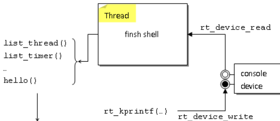
图 12.1: finsh的数据流结构
