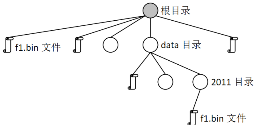
图 13.2: 目录结构
