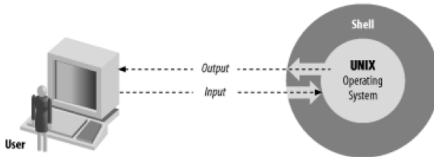
图 12.2: 系统结构图
